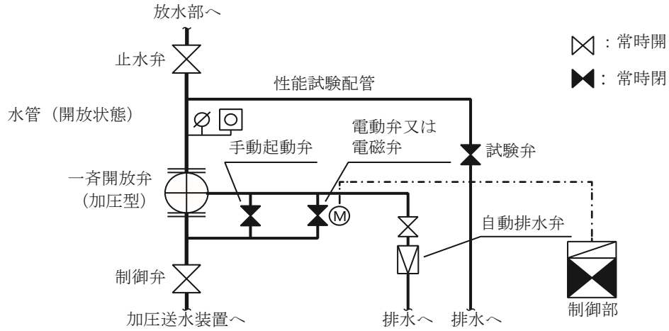
(減圧方式の一斉開放弁等回りの配管例)
